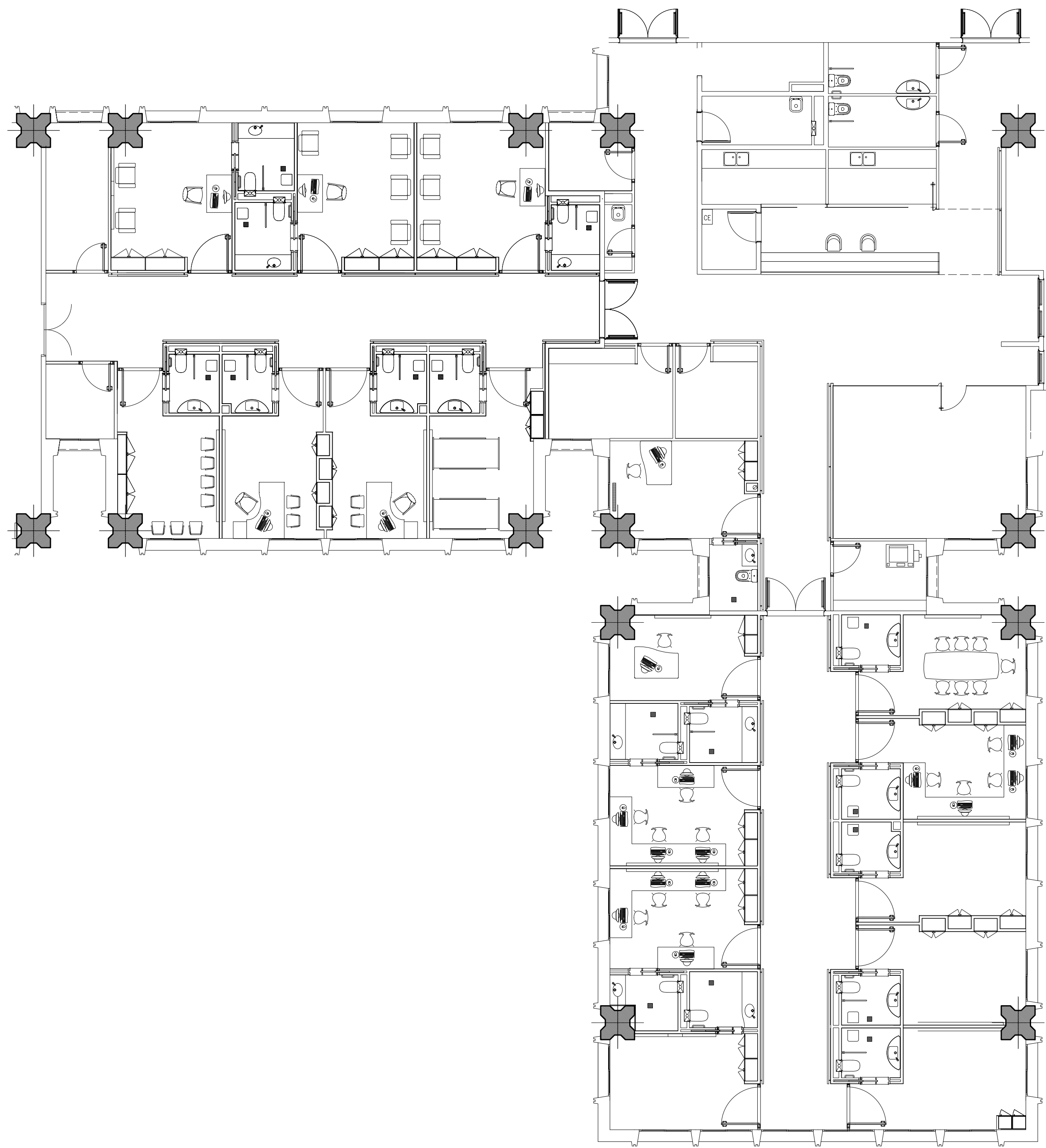
UIC (Fase I) PLANTA 5 S: 714.20 m²
