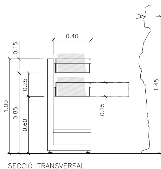
SECCIÓ TRANSVERSAL
