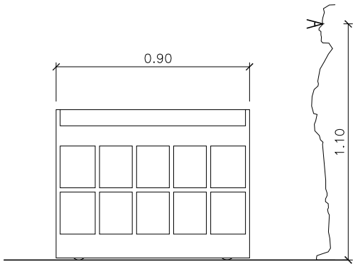
ALÇAT FRONTAL
