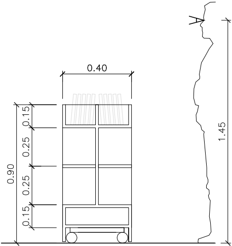
SECCIÓ TRANSVERSAL
