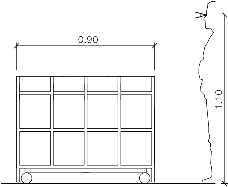
SECCIÓ LONGITUDINAL
