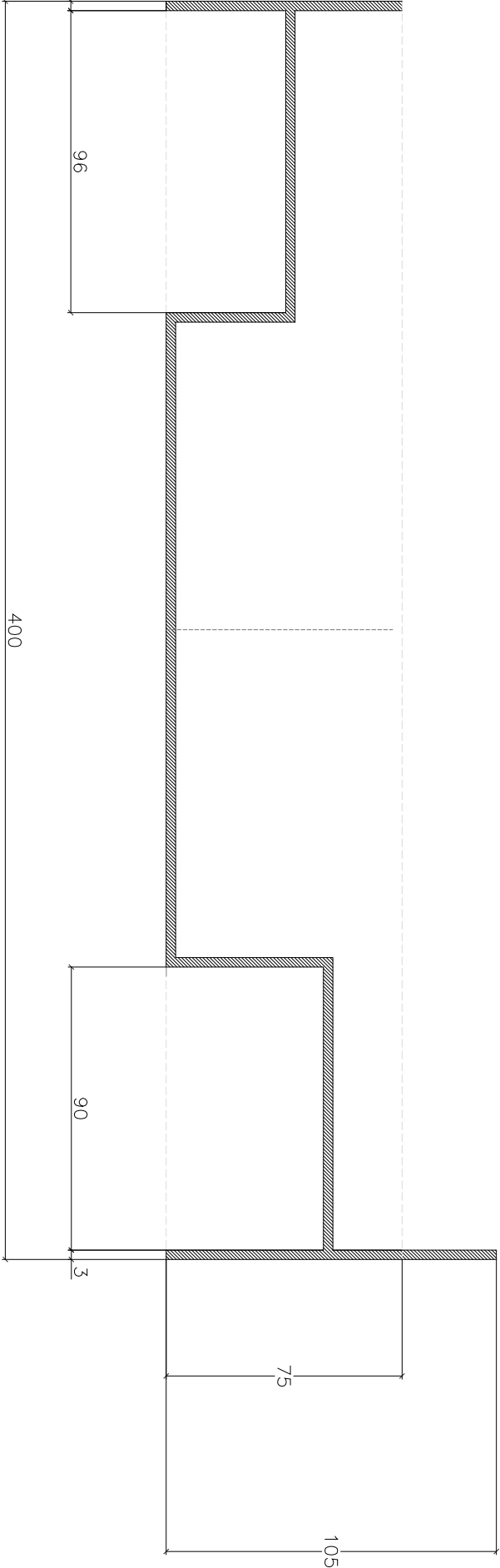
SECCIÓ PLANTA
