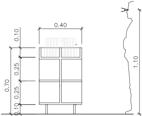
SECCIÓ TRANSVERSAL
