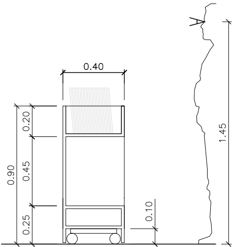
SECCIÓ TRANSVERSAL
