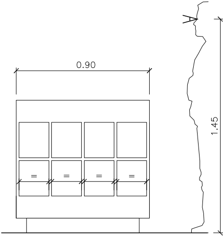
ALÇAT FRONTAL
