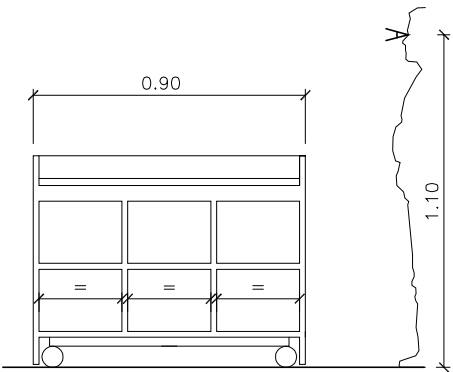
SECCIÓ LONGITUDINAL
