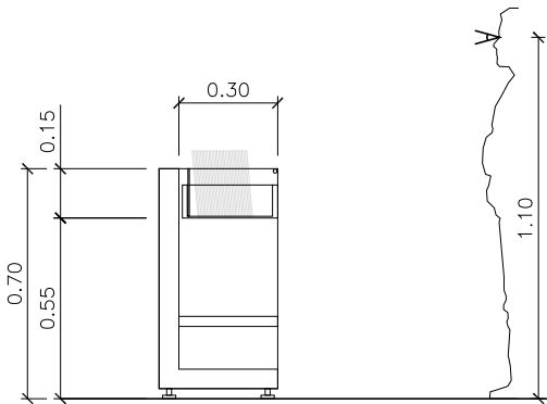
SECCIÓ TRANSVERSAL
