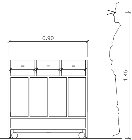
SECCIÓ LONGITUDINAL
