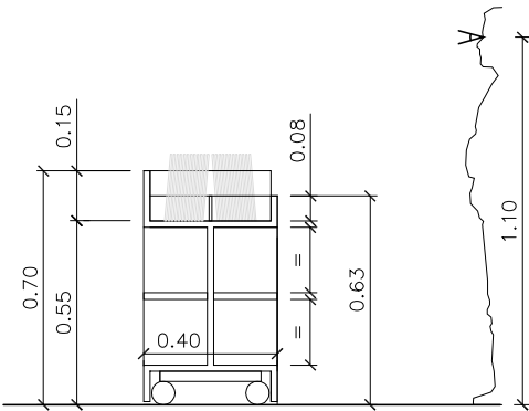
SECCIÓ TRANSVERSAL
