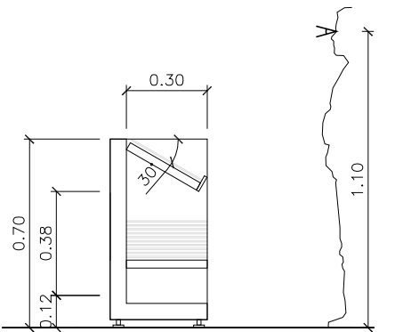
SECCIÓ TRANSVERSAL
