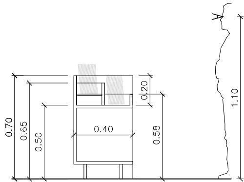
SECCIÓ TRANSVERSAL
