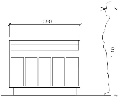
ALÇAT FRONTAL
