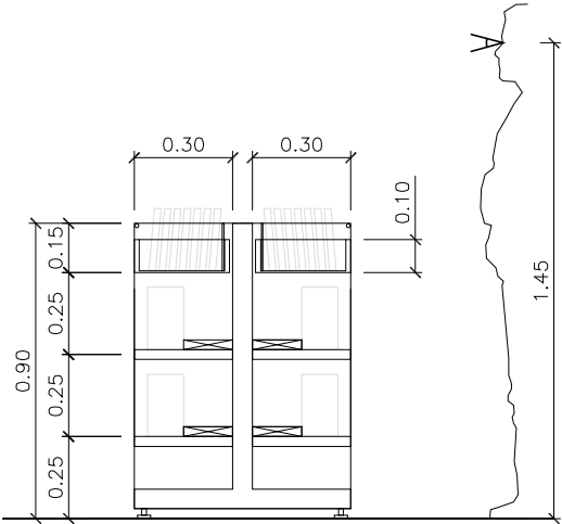
SECCIÓ TRANSVERSAL
