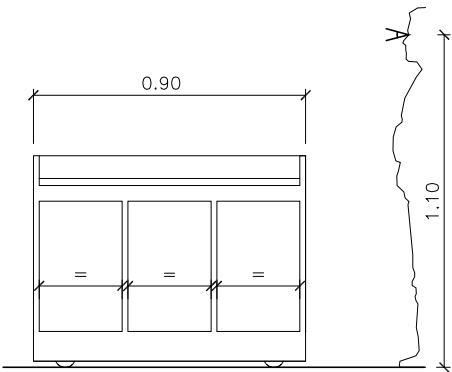
ALÇAT FRONTAL
