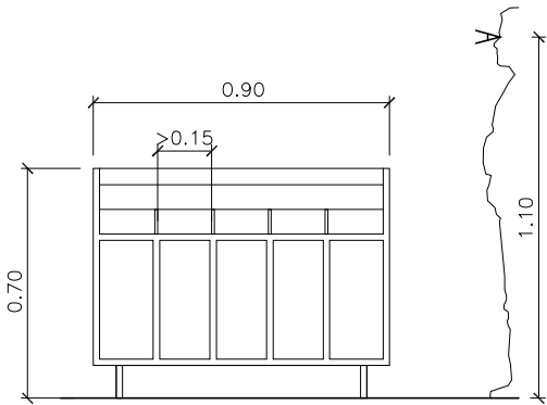
SECCIÓ LONGITUDINAL
