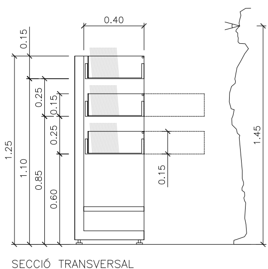
SECCIÓ TRANSVERSAL
