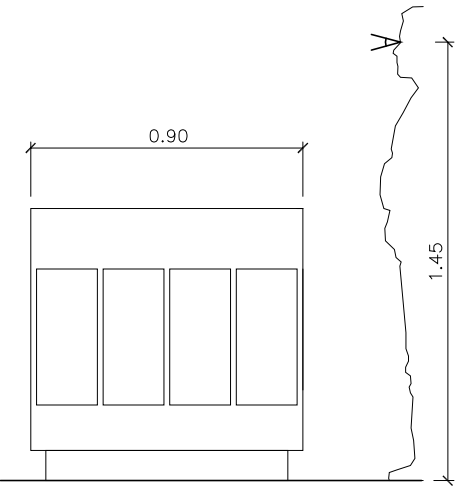
ALÇAT FRONTAL
