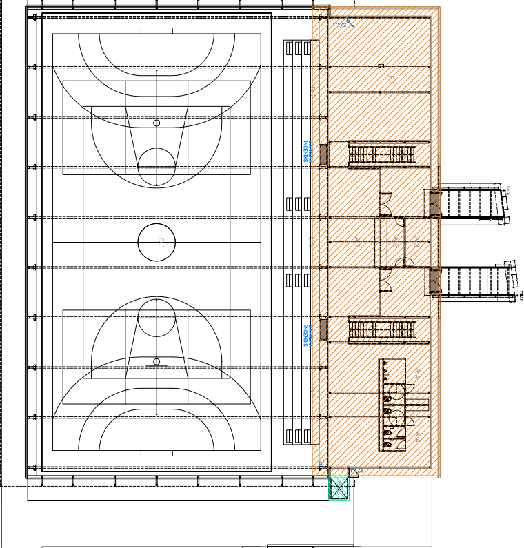
SECTORS INCENDI PLANTA PRIMERA
