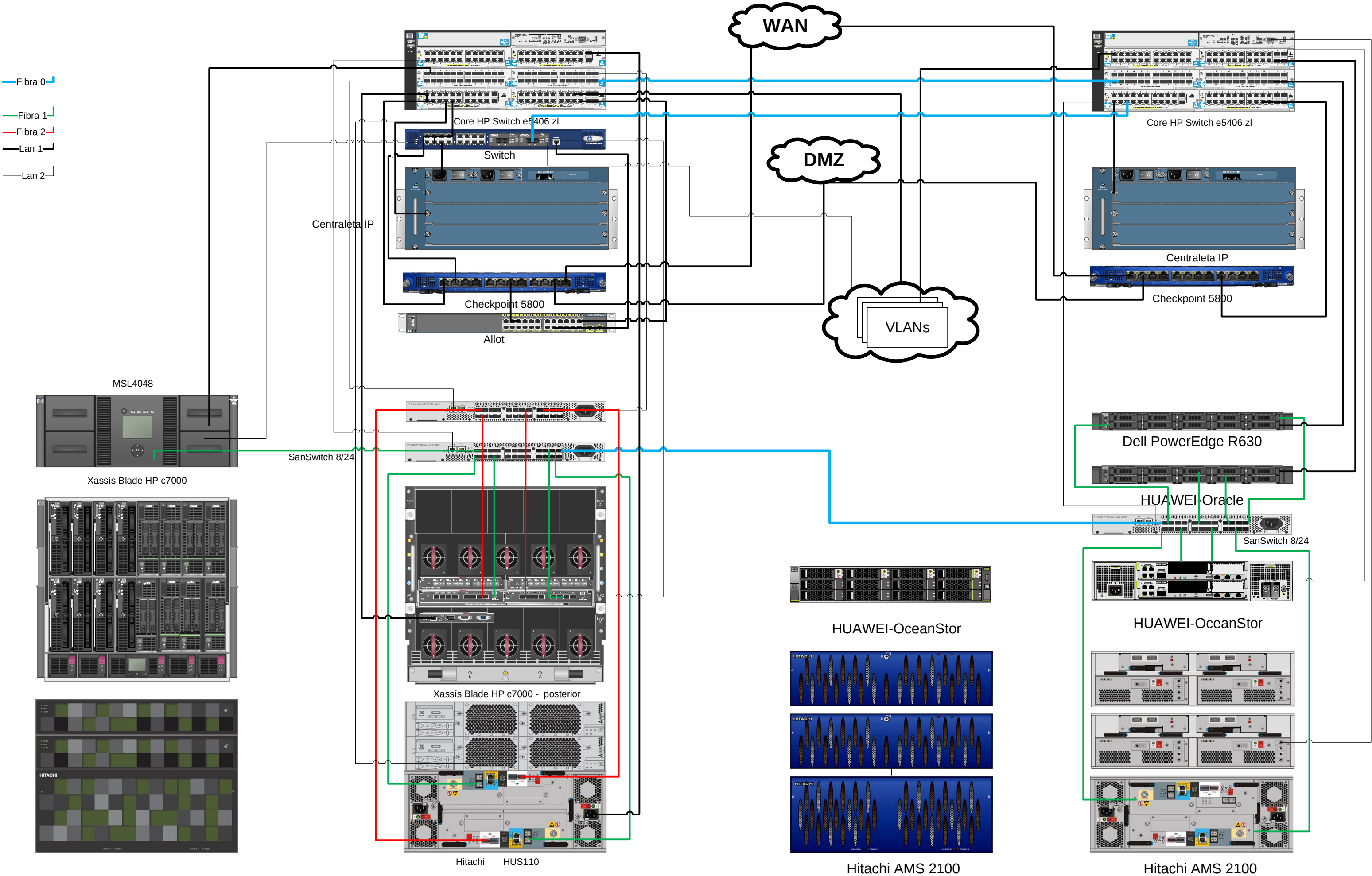
Esquema bàsic CPD Ajuntament de Sant Cugat del Vallès
