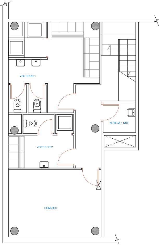
PLANTA SOTERRANI
