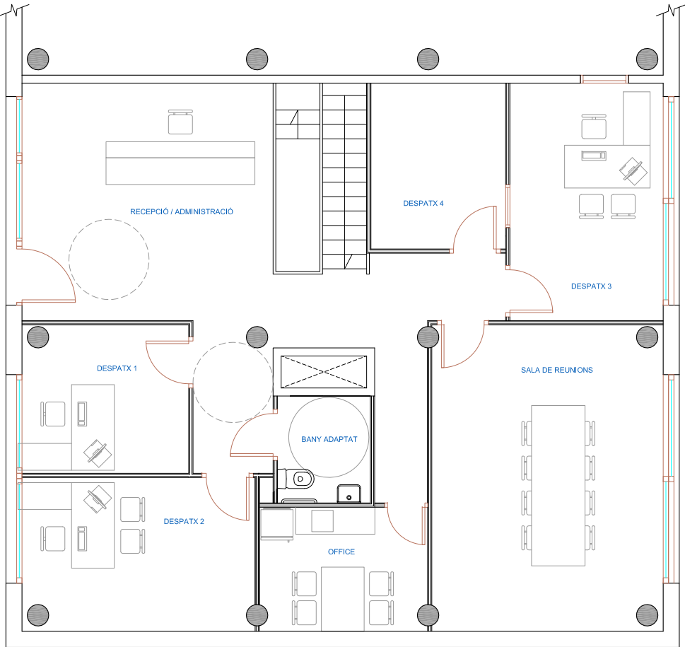
PLANTA BAIXA
