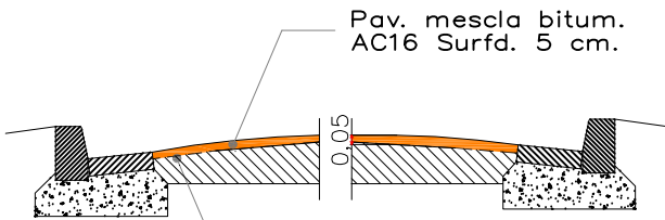
MILLORA 2: ASFALTAT C./ PERELLÓ I PAS ELEVAT. PRIORITAT D'EXECUCIÓ DELS TRAMS: DE L'1 AL 6 EN AQUEST ORDRE.
