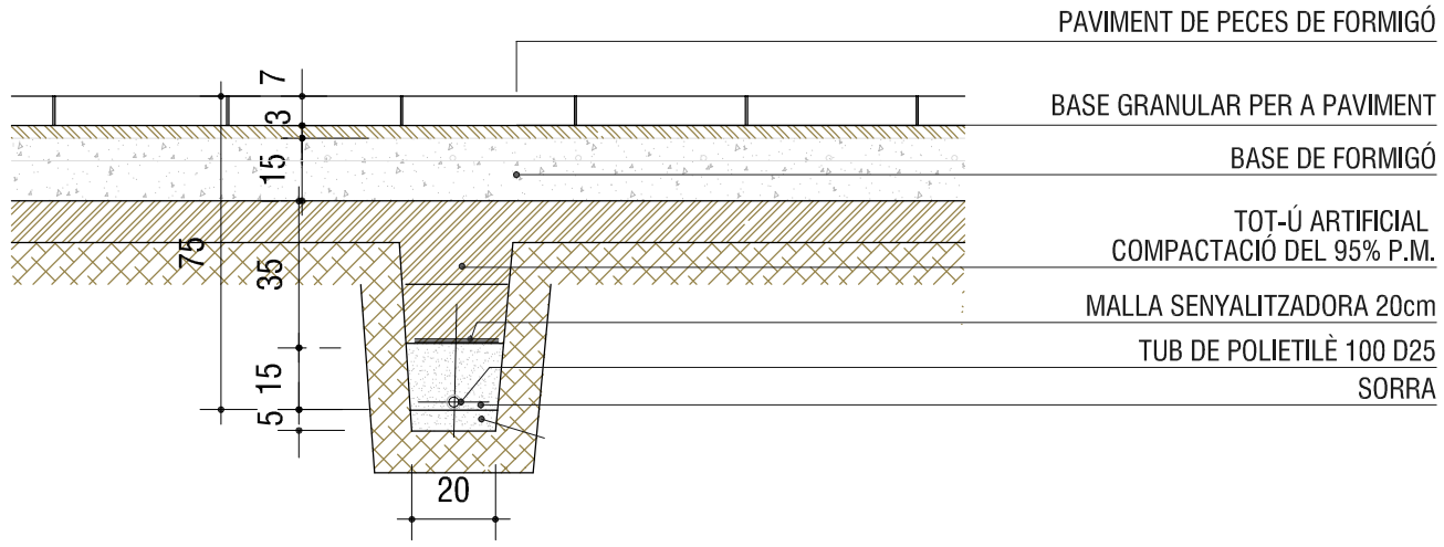
DETALL RASA CANALITZACIÓ AIGUA POTABLE
