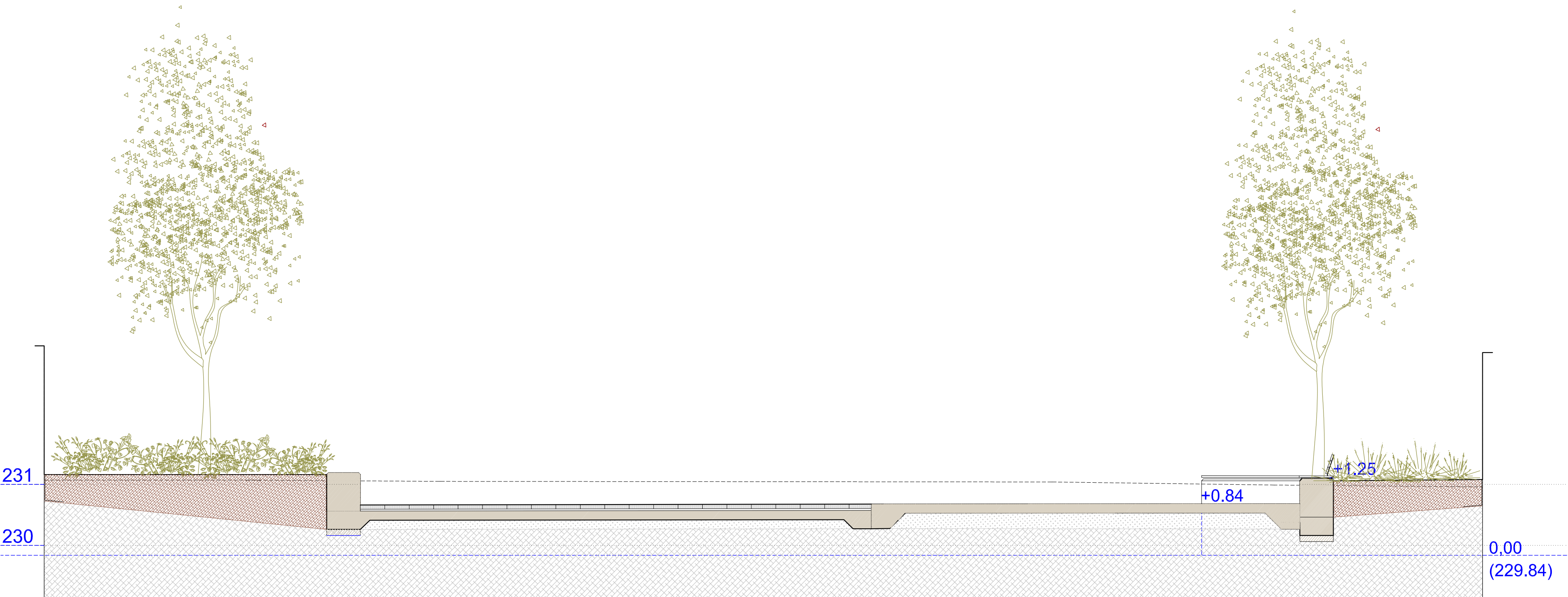
secció 7 (e:1/100 dinA3 1/50 dinA1)
