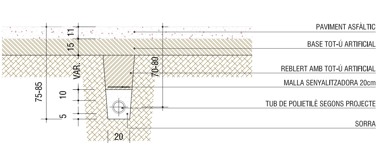
DETALL RASA CANALITZACIÓ AIGUA SOTA CALÇADA
