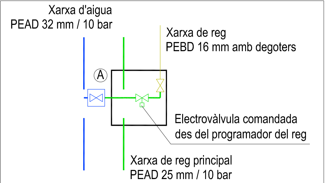
DETALL ARQUETA PER A DISTRIBUCIÓ DE LA XARXA DE REG
