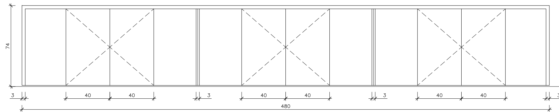
ALÇAT
