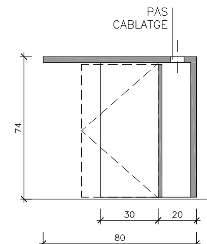
SECCIÓ
