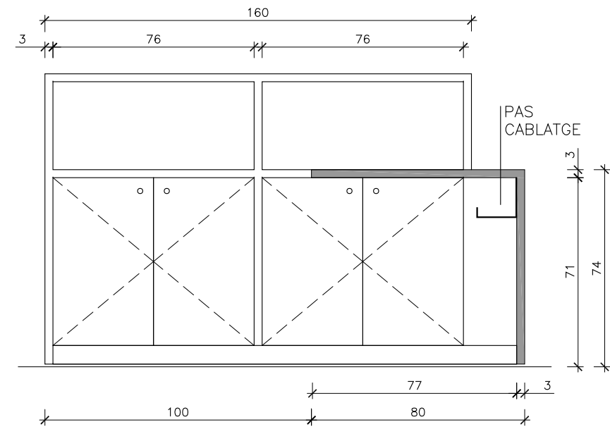
SECCIÓ V1-V1'
