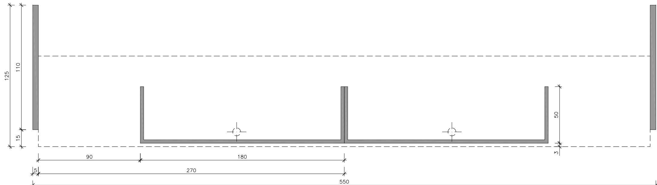
PLANTA SECCIONADA H=40
