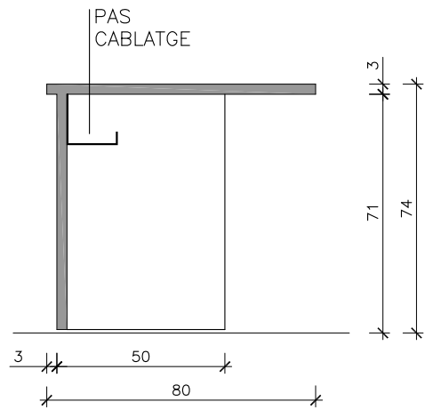
SECCIÓ V2–V2’
