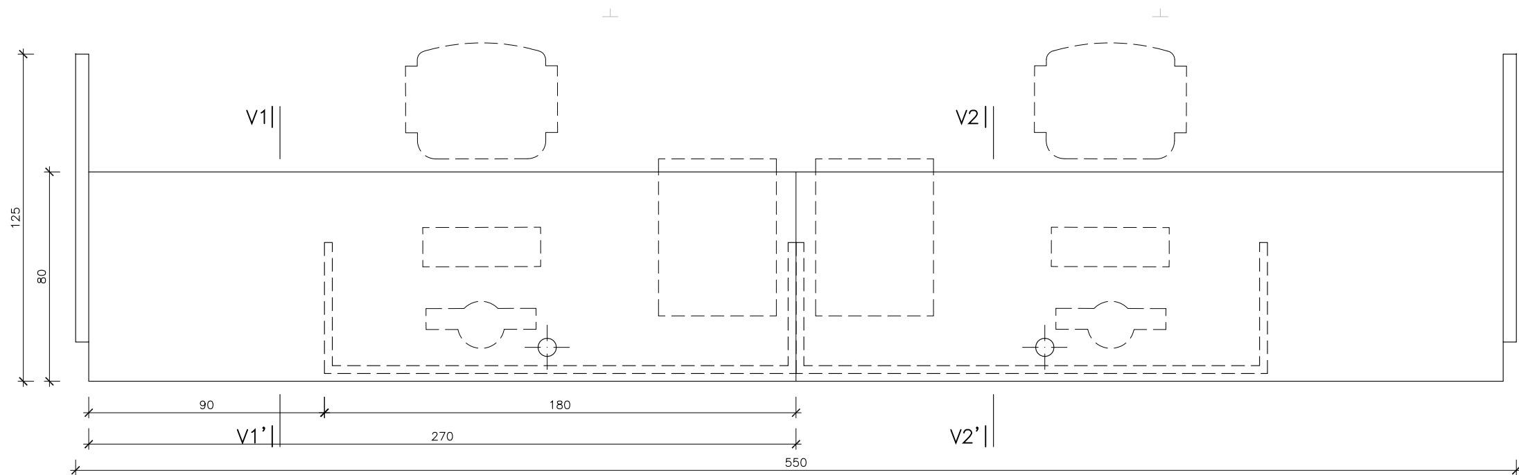
PLANTA
