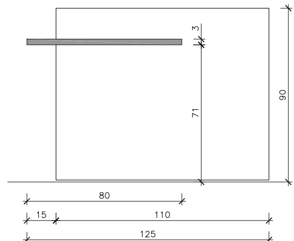
SECCIÓ V1–V1’
