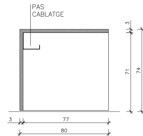
SECCIÓ V2-V2'
