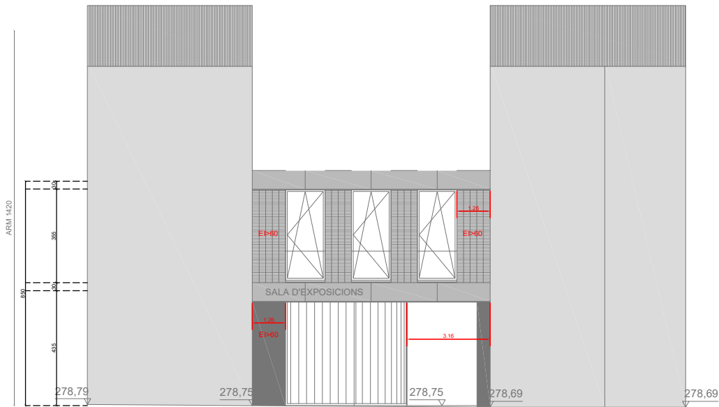
ALÇAT A CARRER SALVADOR VANCELL
