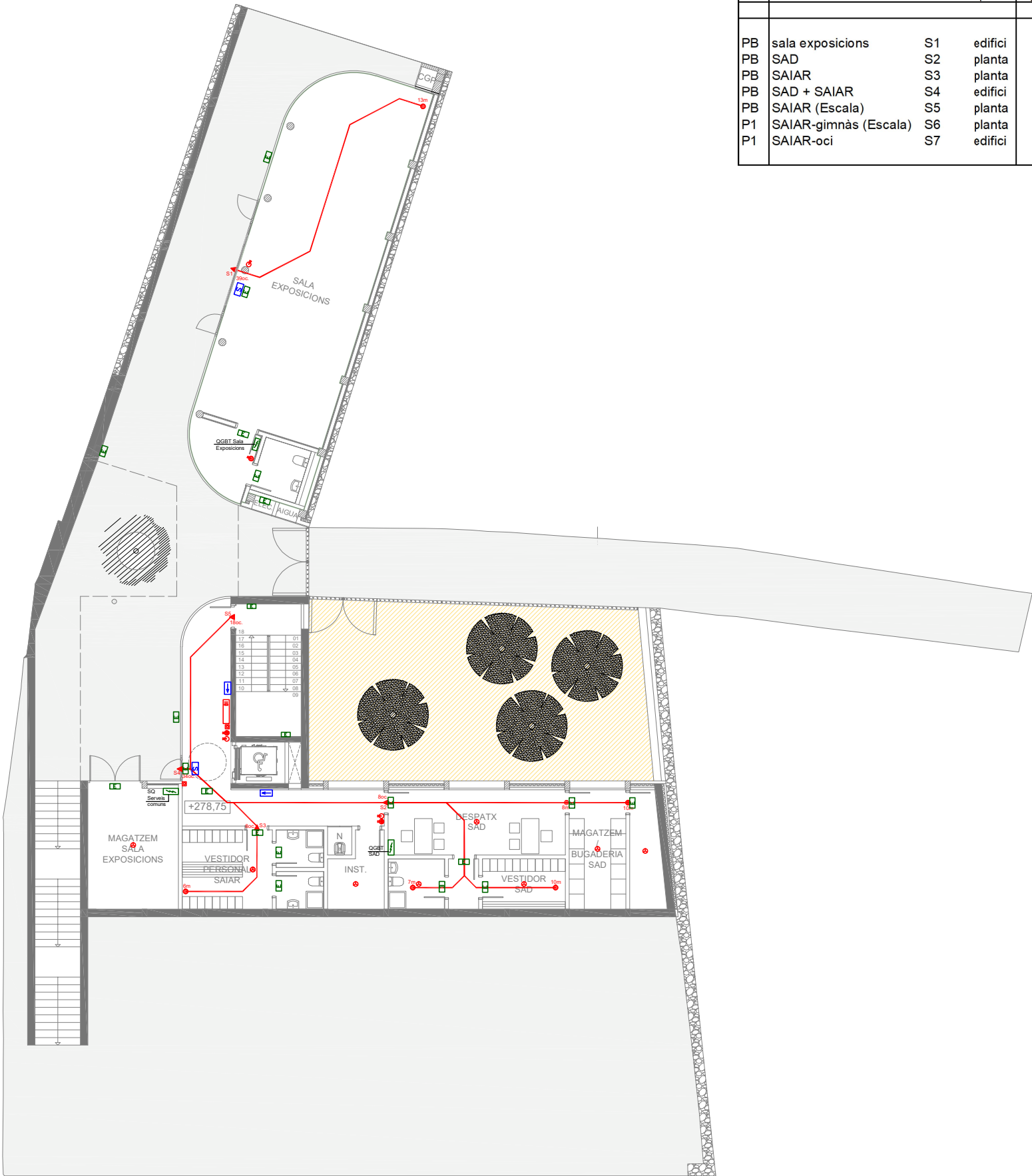
Planta baixa: Protecció contra incendis
